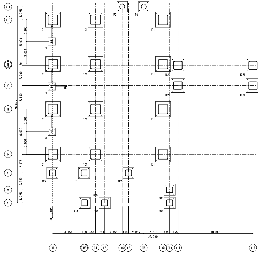
アンカープラン 柱 断面1/30 特記なきP.L.下地は G.L.±0 レベルはG.L.を基準
